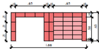
DET. 1 CHURRASQUEIRA - PLANTA BAIXA 01 | ESC: 1:25
