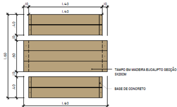
DET. 2 MESA - PLANTA BAIXA
